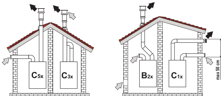
fig. 8 - Ejemplos de conexión con tubos separados ( ← = aire / → = humos )
